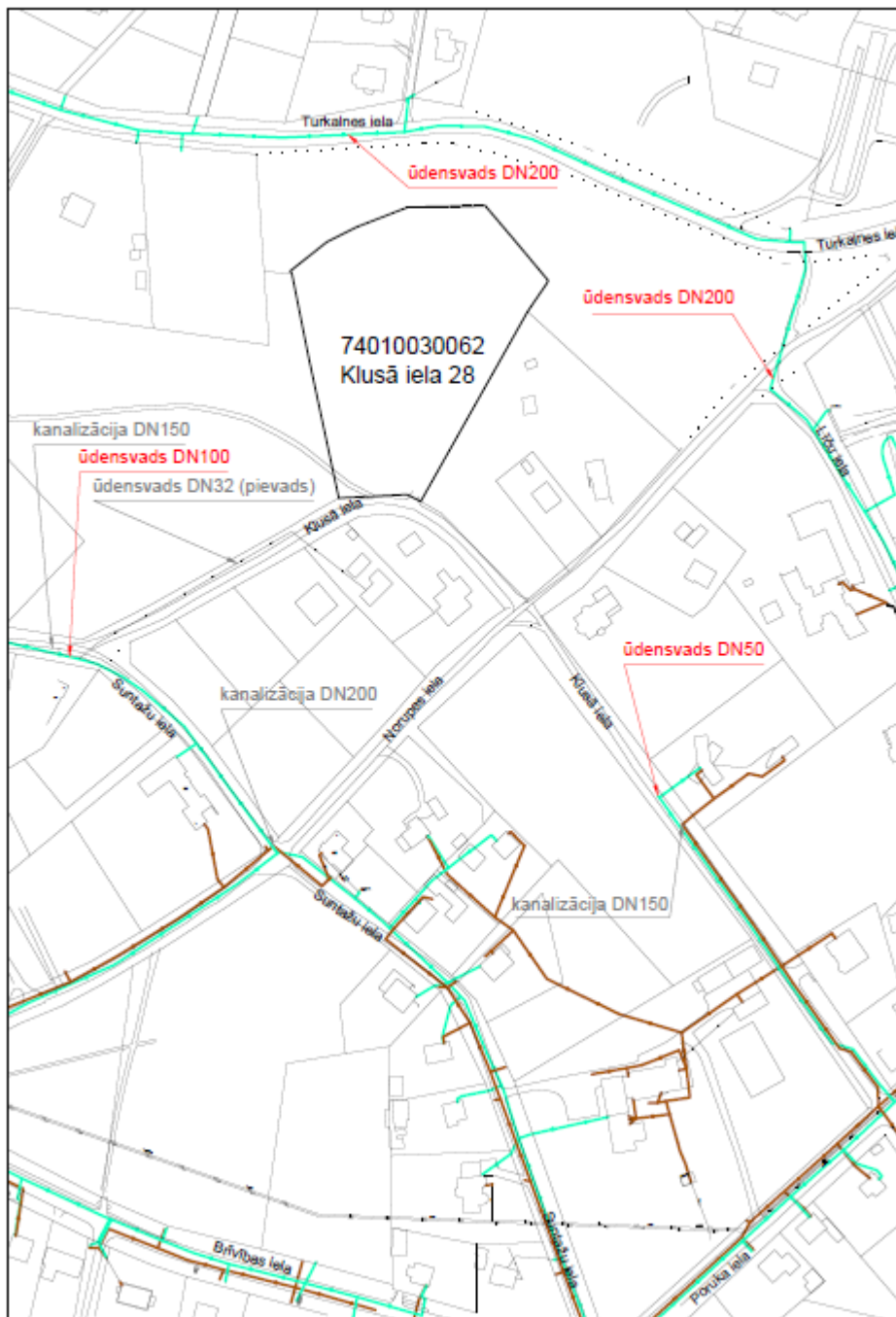
15. attēls. Esošā centralizēto ūdensapgādes un sadzīves kanalizācijas tīklu shēma. Pielikums Aģentūras 21.07.2023. tehniskajiem noteikumiem Nr.1-10/133.
